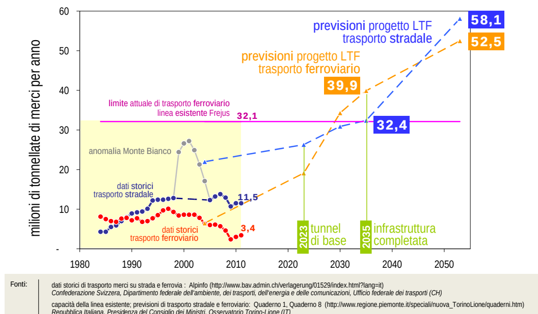
Fig. 2 – Traffico merci nel corridoio transalpino della Valle di Susa : dati storici vs previsioni
