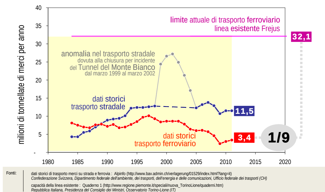
Fig. 1 – Traffico merci nel corridoio transalpino della Valle di Susa : dati storici vs capacità
